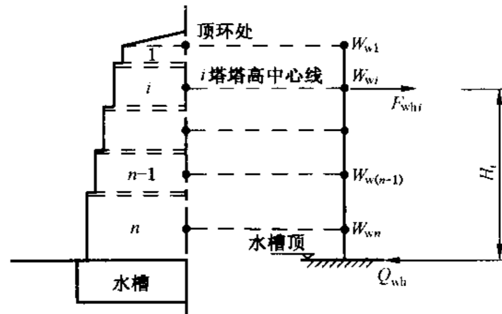
图 7.4.1 湿式罐结构计算简图
