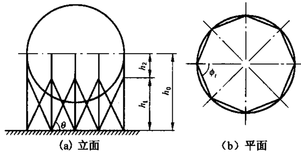
图 7.2.3 球罐简图
